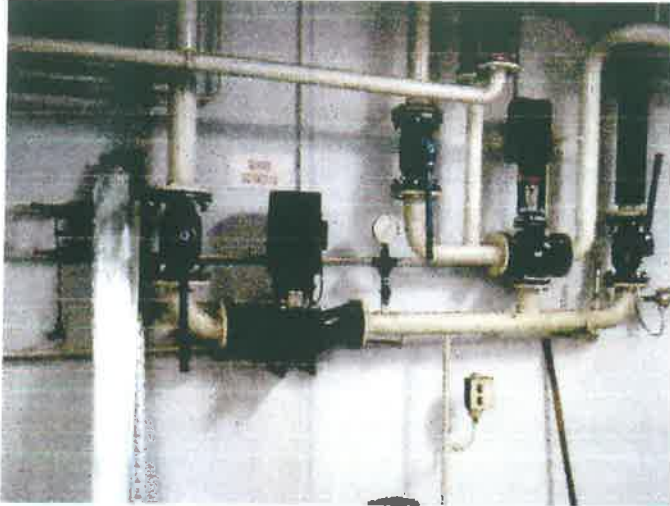
Hőhasznosító rendszer:
